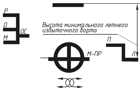
Рис. 14.4.2 Грузовая марка на судах класса «М-ПР» с минимальным надводным бортом
